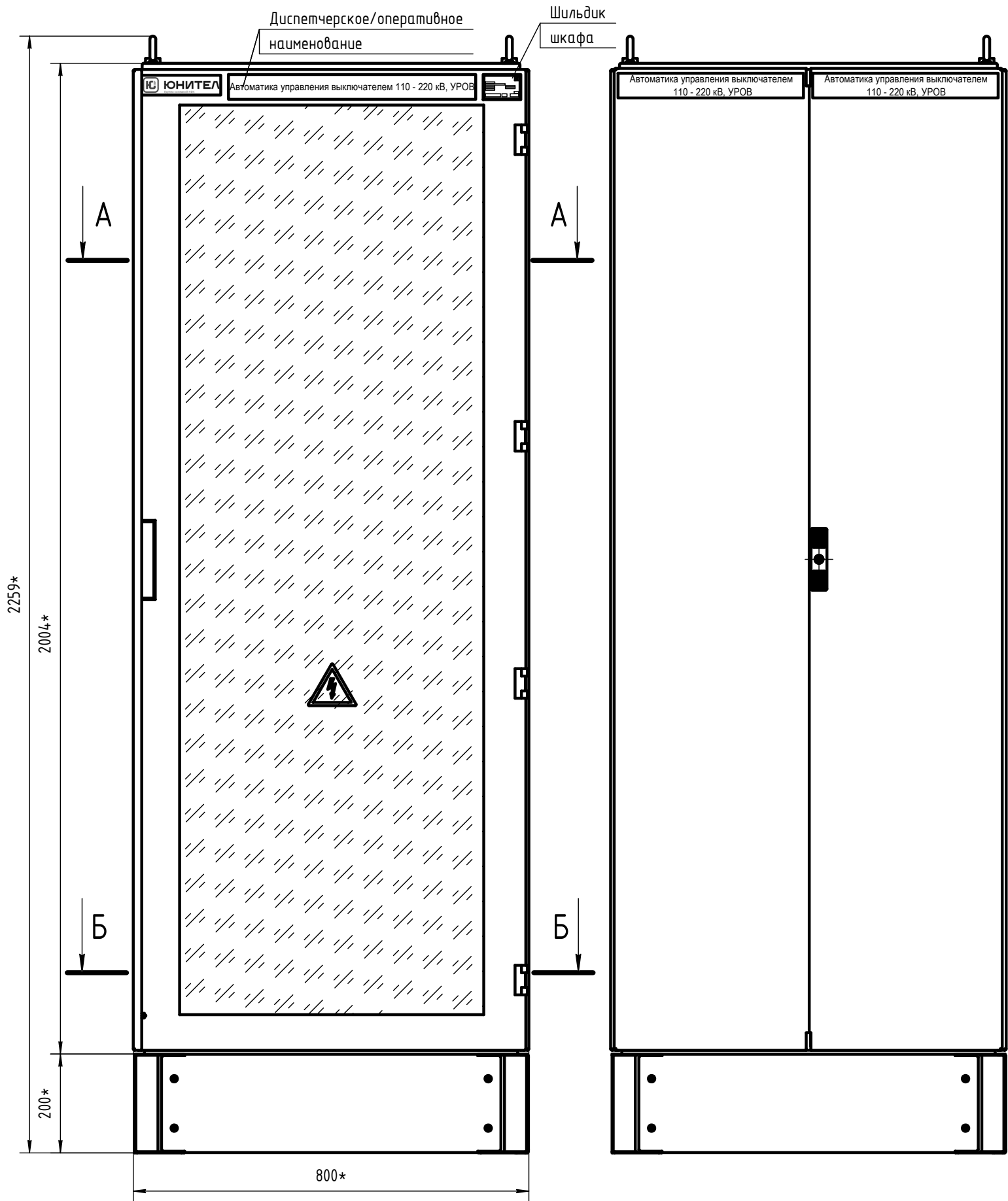
Вид сзади
