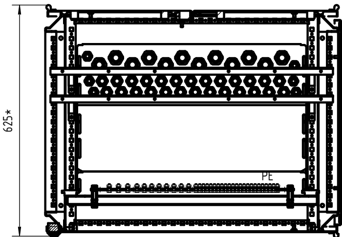
Б-Б
